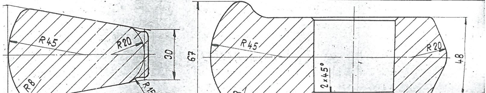
PRIEREZ G-G POOTOČENÝ
