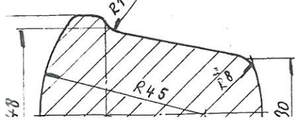
PRIEREZ V-V POOTOČENÝ
