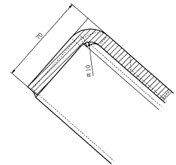
SCHNITT D-D M 1:1
