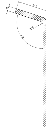
SCHNITT C-C M 1:1
